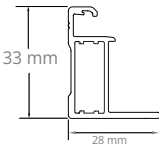
PROFIL DU GRAND CÔTÉ
