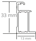
PROFIL DU PETIT CÔTÉ
